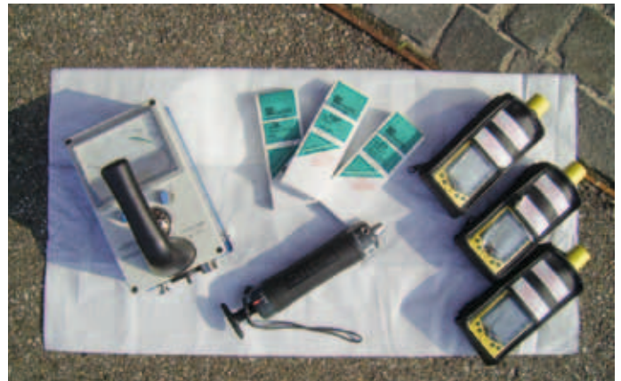
Messgeräte zum Messen von Gas- und Dampfgemischen.
